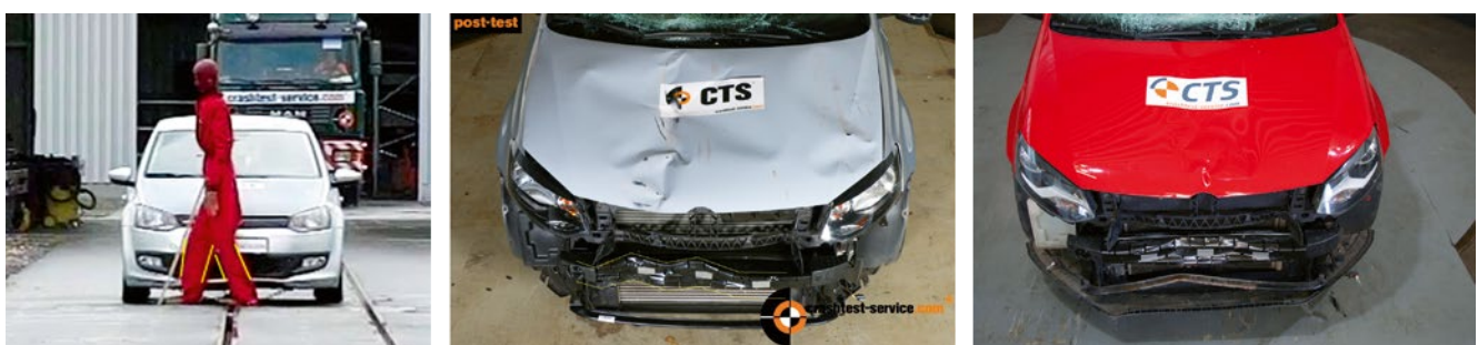
BILD 8: Schrittstellung beim Anfahren des konventionellen Dummys (links) und daraus resultierende Querträgerverformung (Mitte) bei v=70 km/h; Vergleich der Frontbeschädigung beim Anprall gegen einen Biofidel-Dummy (rechts)
